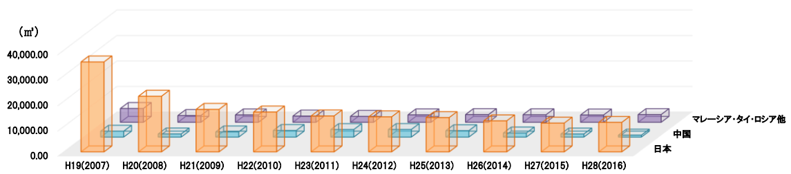
(13) 生産国別（造作用集成材）の年別格付数量
