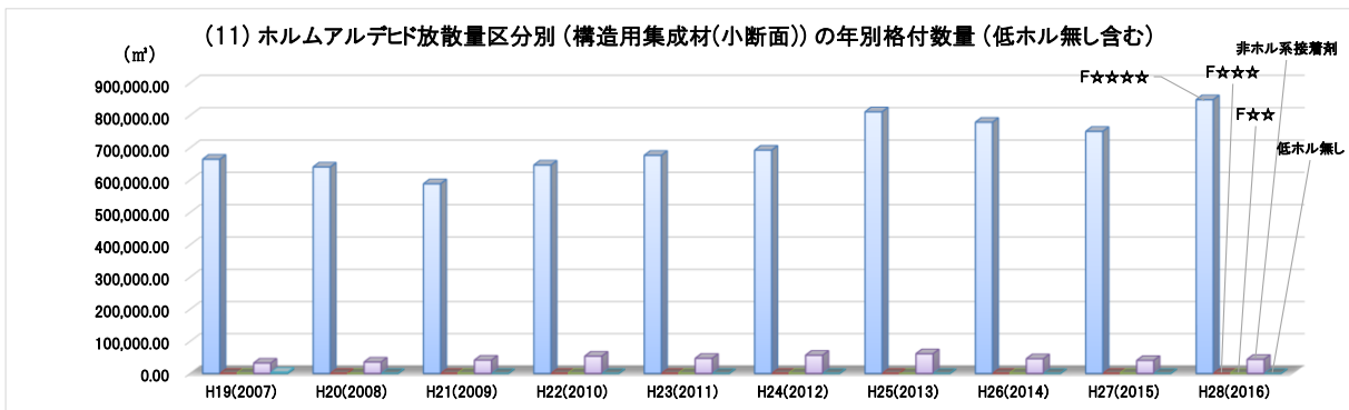
(11) ホルムアルデヒド放散量区分別（構造用集成材（小断面））の年別格付数量（低ホル無し含む）
